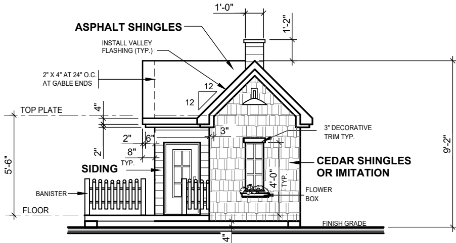
RIGHT ELEVATION
